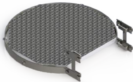
Plataforma fixa com chapa ondulada em alumínio REF: 100146
